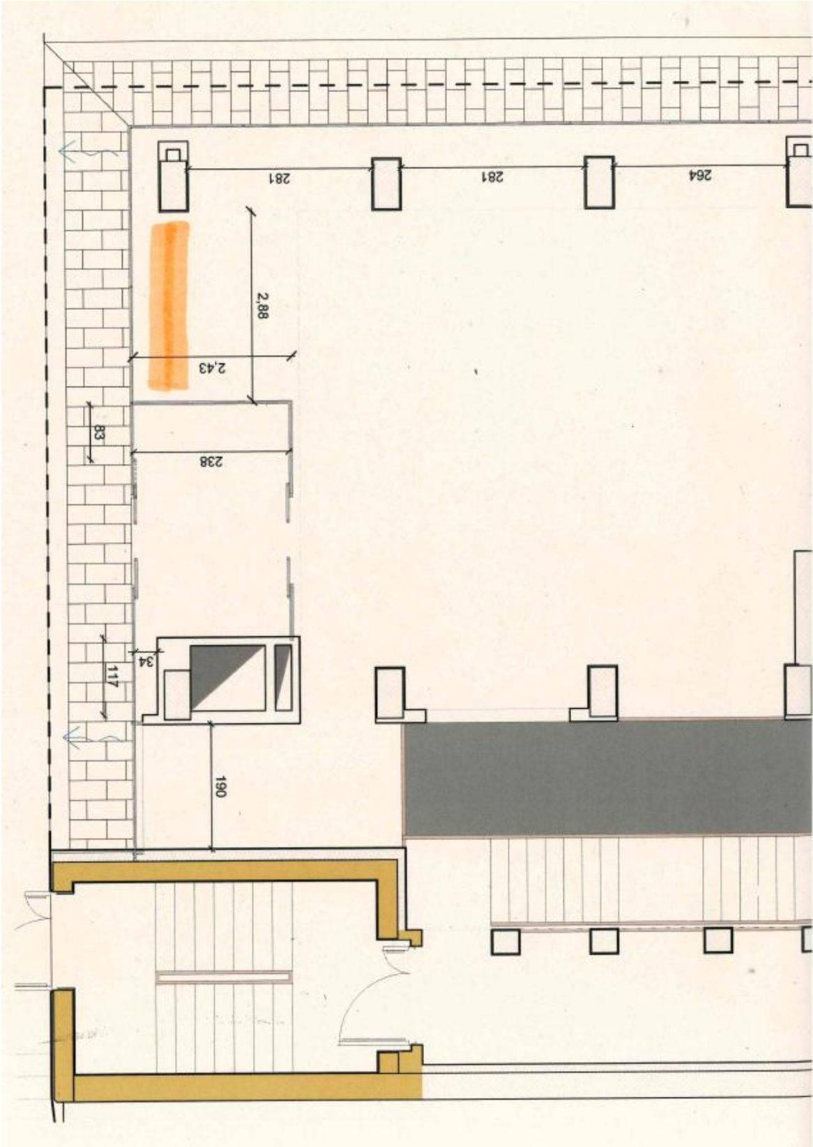
FIGURA 3 PIANTA PIANO TERRA ZONA A SINISTRA DELL'ENTRATA
